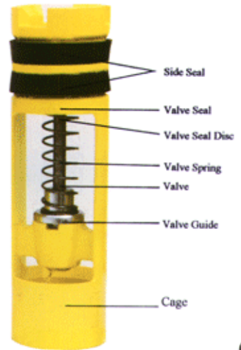
Piston Type
